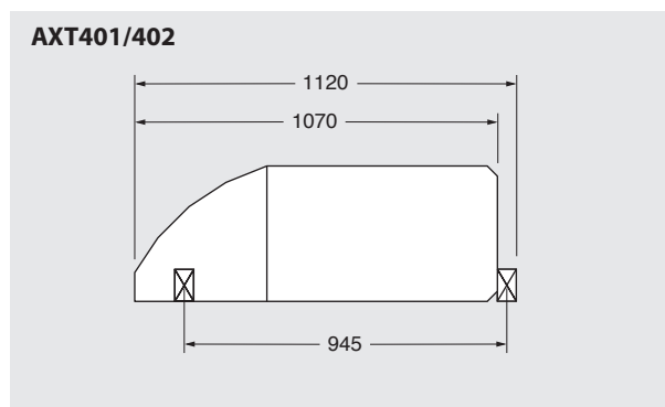
Dodatkowy dyfuzor AXT401/402
